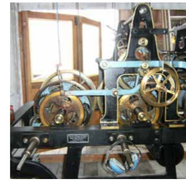
Auslösen des Stundenschlag
