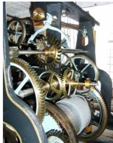
Ankerhämung des Gehwerks
