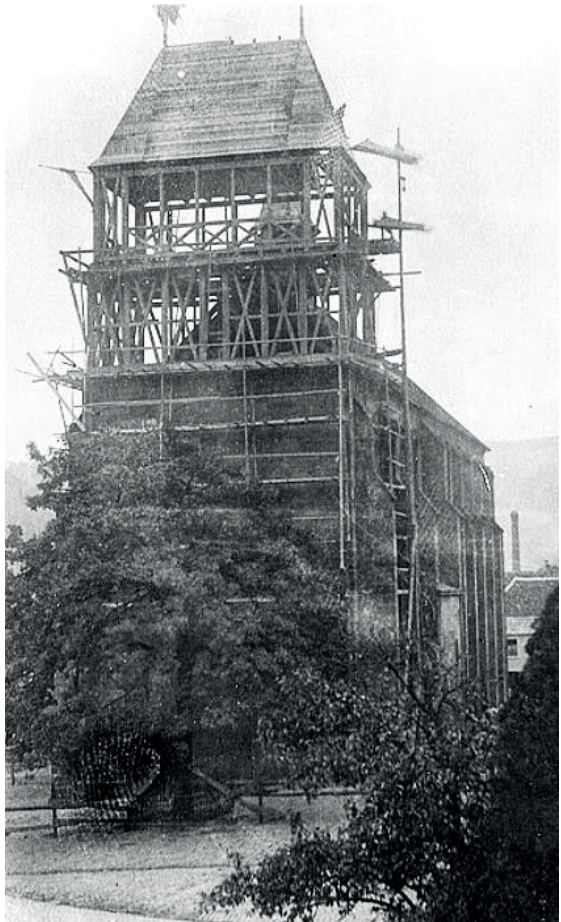
Aufbau der Glockenstube an der Westseite der Kirche
